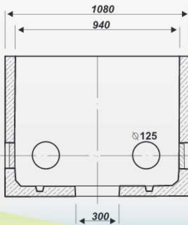
Przekrój podłużny
